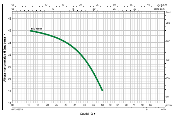
CURVAS Y DATOS DE PRESTACIONES
